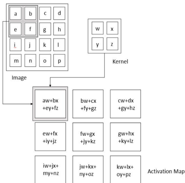
Fig. 3. Convolution Layer
