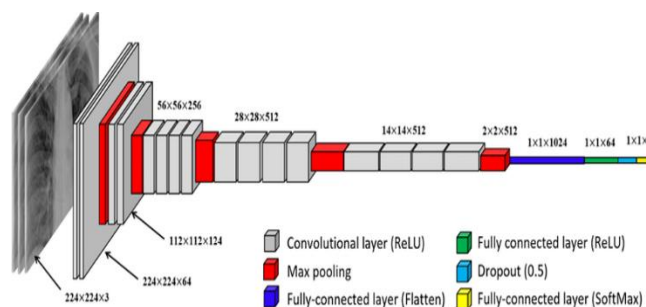
Fig. 6. vgg-19
